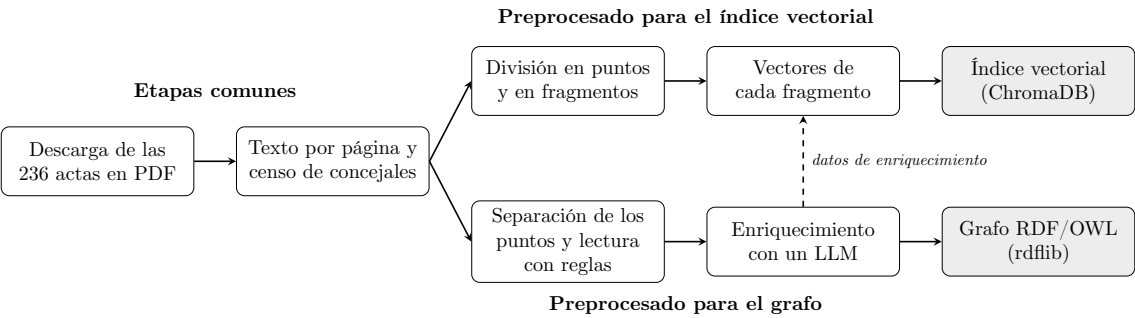
Figura 12: Esquema del preprocesado: etapas comunes y proceso específico de cada estructura de datos
