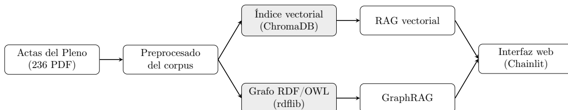
Figura 5: Arquitectura general: dos estructuras de datos sobre los mismos documentos
