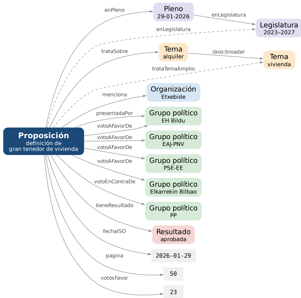
Figura 7: Selección de los triples de una proposición del grafo. Las flechas discontinuas son triples materializados por el razonador y los rectángulos grises, valores literales
