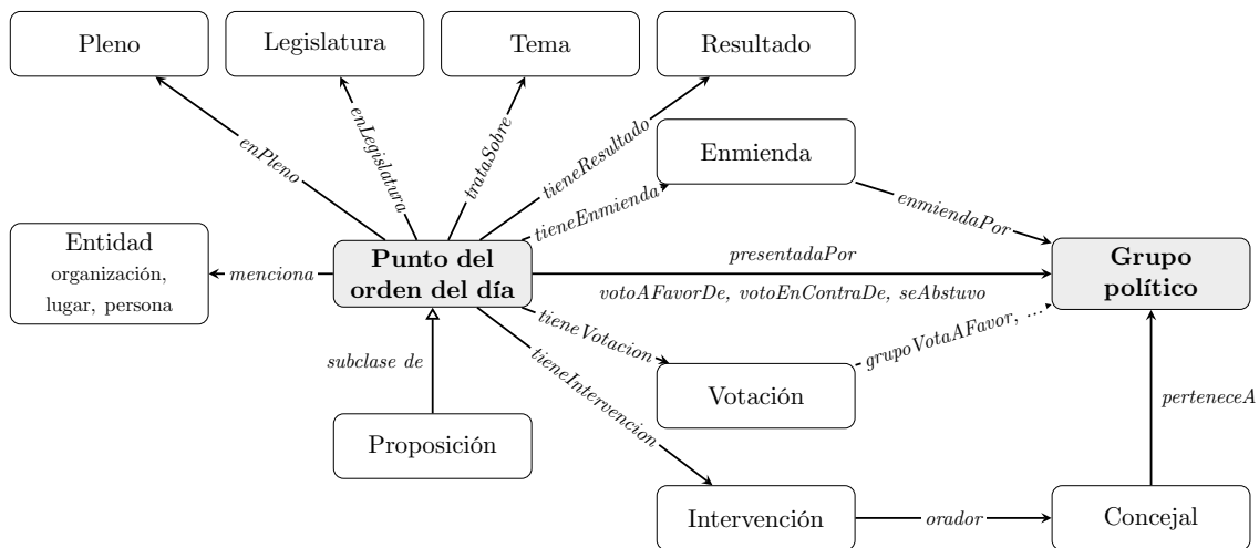
Figura 6: Clases principales de la ontología y propiedades que las relacionan
