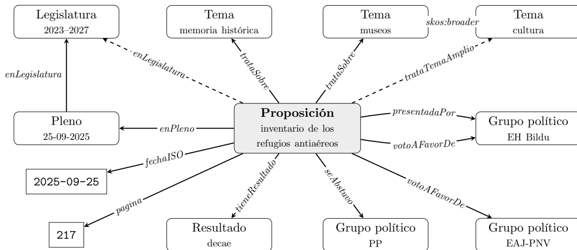
Figura 7: Selección de los triples de una proposición del grafo. Las flechas discontinuas son triples materializados por el razonador y los rectángulos, valores literales
