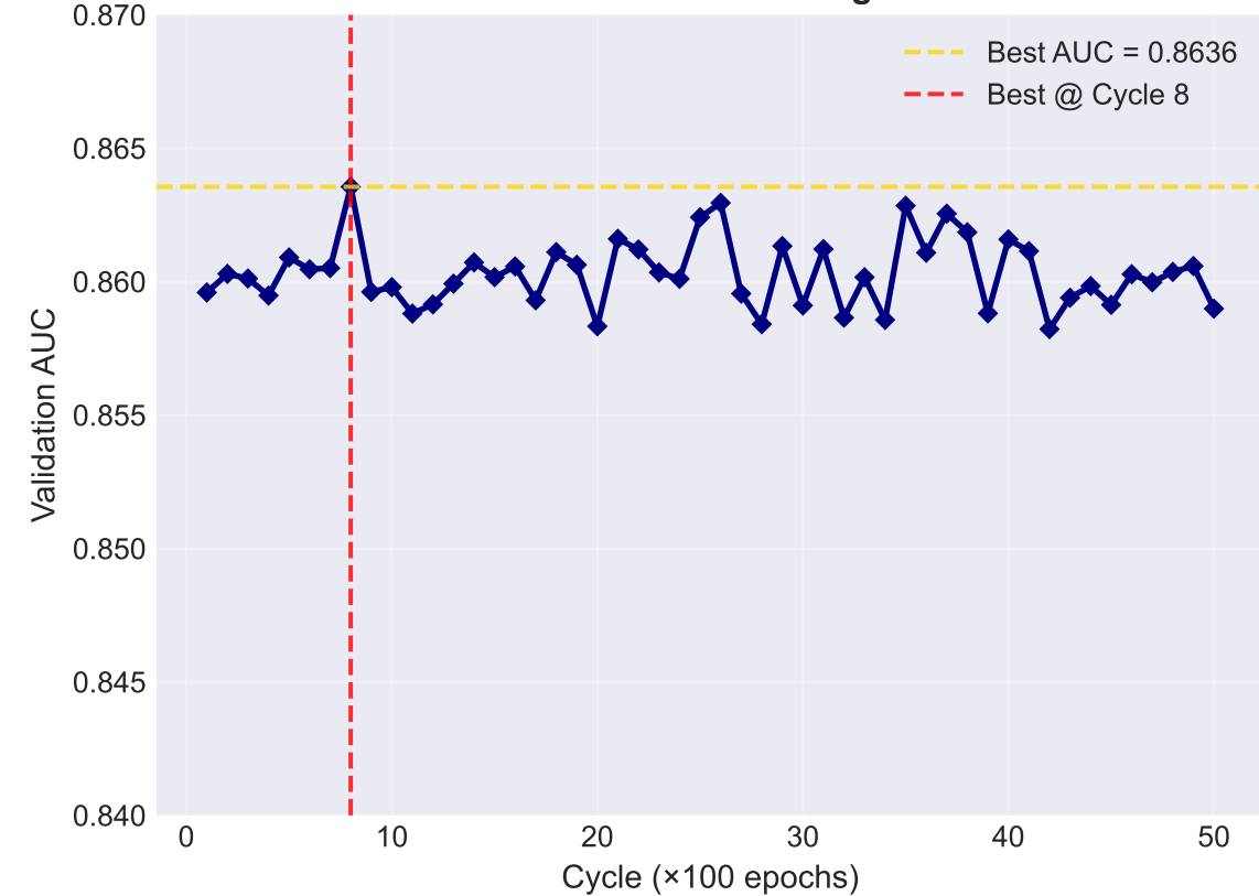
Validation AUC Convergence
