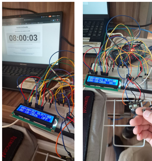
Figura 1: Protótipo em operação: alinhamento inicial com referência visual e indicação de alarme habilitado. Fonte: registro do autor, 08/10/2026.
