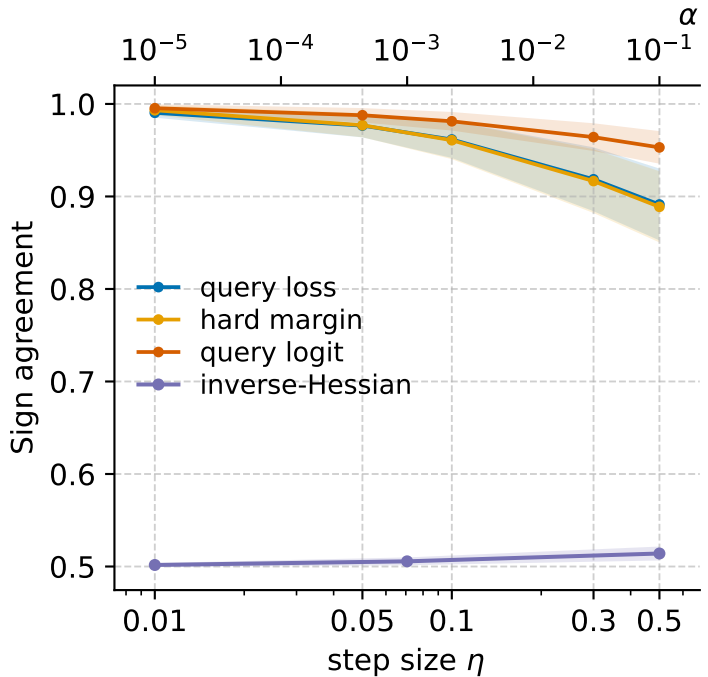
(d) CIFAR-10
