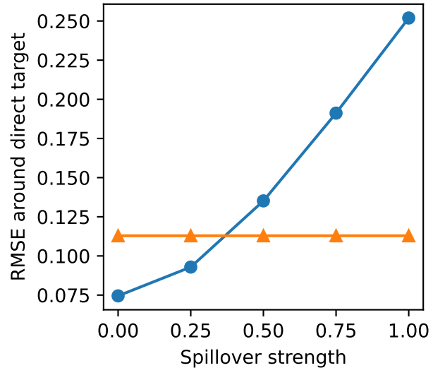
B. Bias--variance tradeoff
