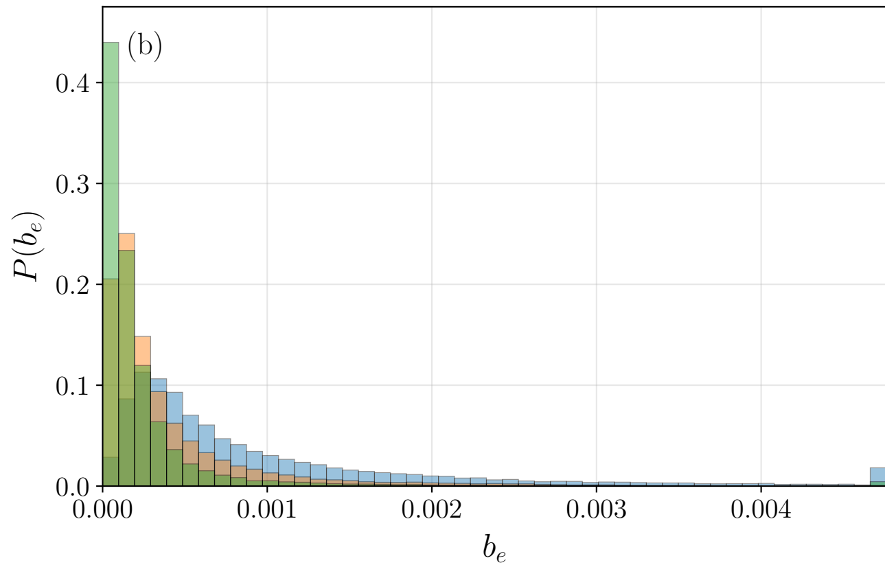
Edge betweenness
