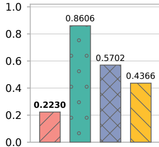
MAE ↓
