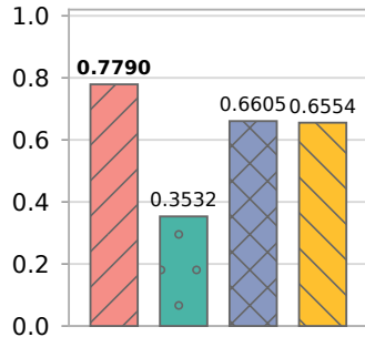
Macro-F1 ↑
