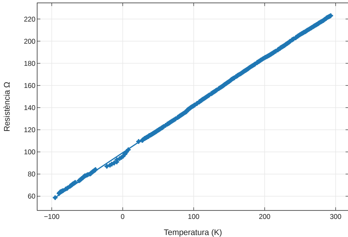
Resistència ( \Omega ) en funció de la temperatura (K)
