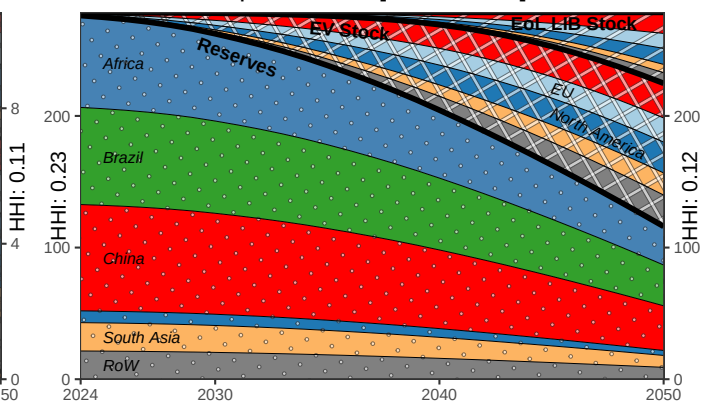
(d) Natural Graphite Stock [million tons]
