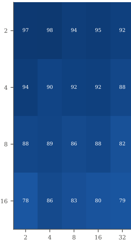
mlp
