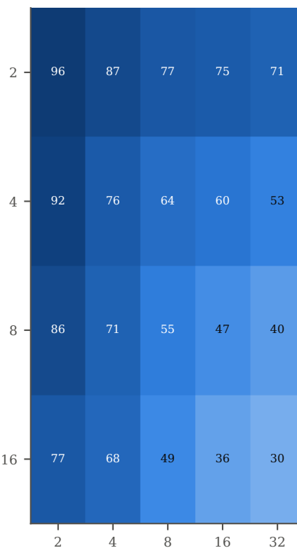
quadratic
