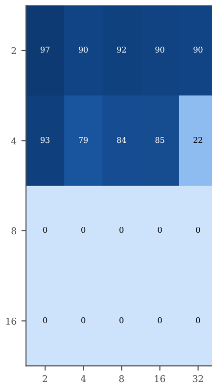
polar3
