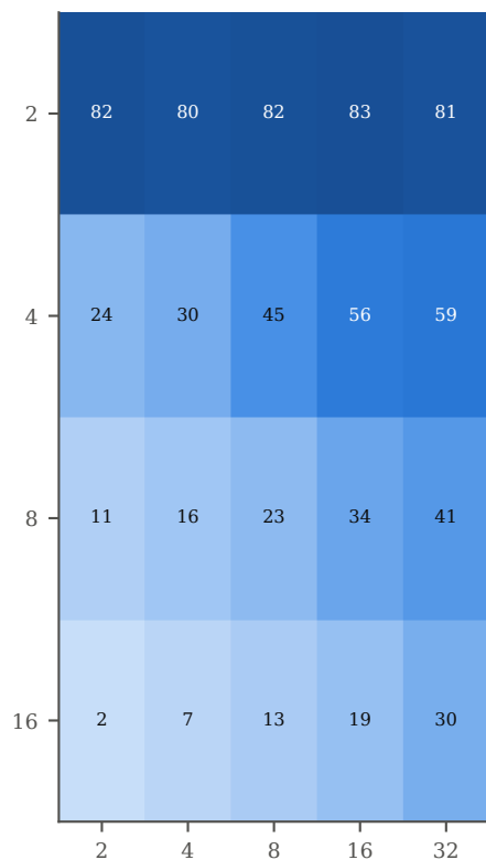
polar8
