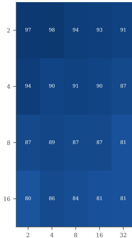
polar3
