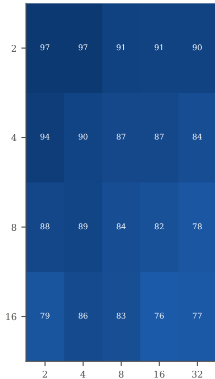
polar8
