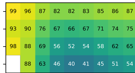
mode F1
