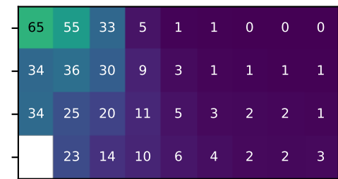
hallucination F1
