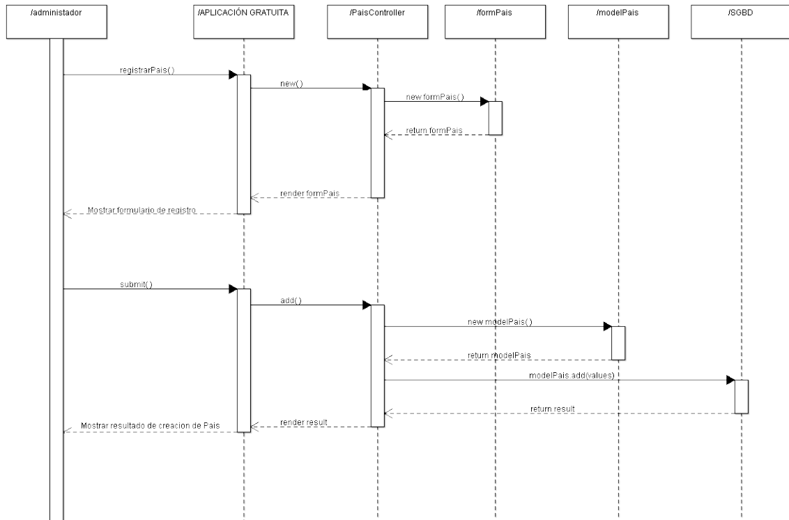
Figura 7.1: Ejemplo de diagrama de secuencia
