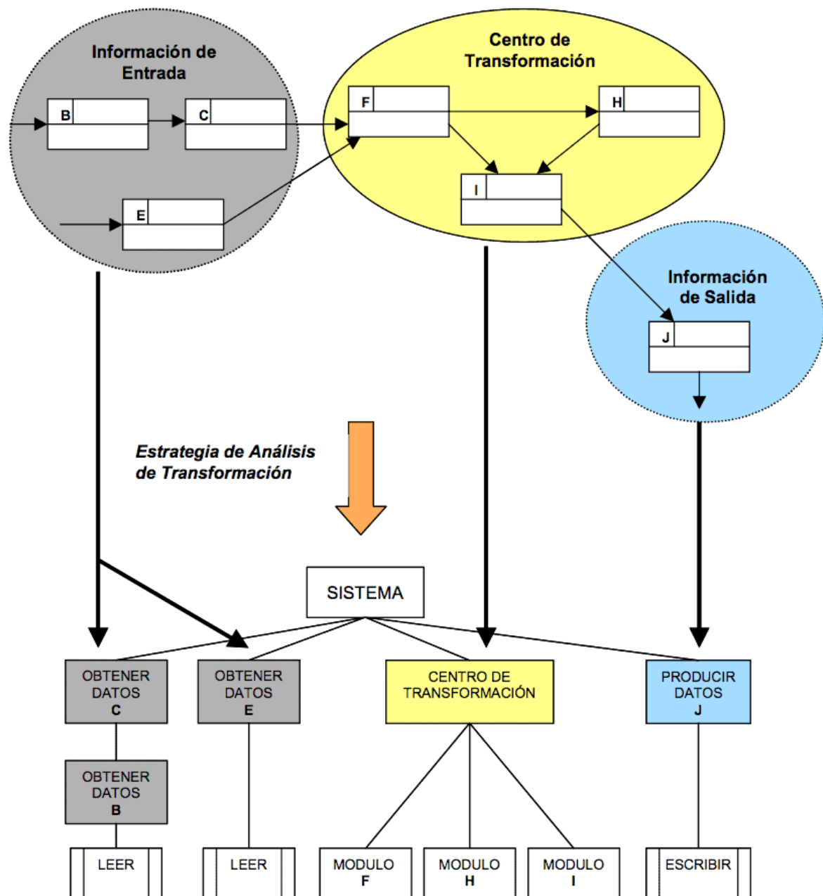
Figura 13.4: Estrategia de Diseño usando Análisis de Transformación
