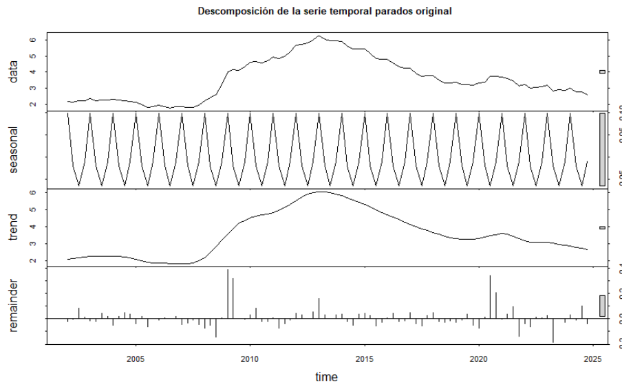
Gráfico 7.3.1: Descomposición de la serie de parados original, y_t .
