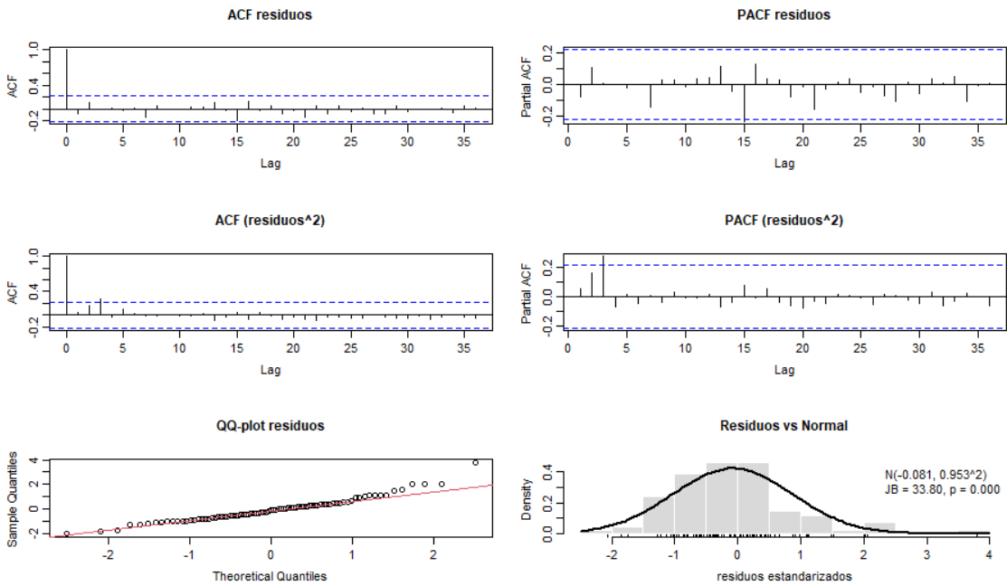
Gráfico 7.3.7: Cuadro resumen de diagnóstico de los residuos del modelo 7.3.4. Nota: la primera fila muestra la ACF y PACF de los residuos; la segunda, la de los residuos al cuadrado; la tercera, el
