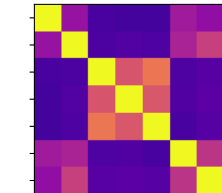
EAP-IG
