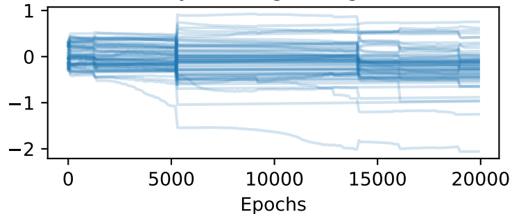
Layer 1 Edge Weights
