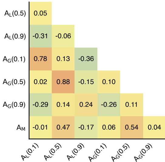
(d) Jaccard, \sigma_R = 0.05
