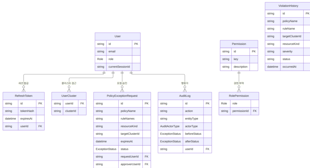
그림 3. 데이터 모델(ERD)
