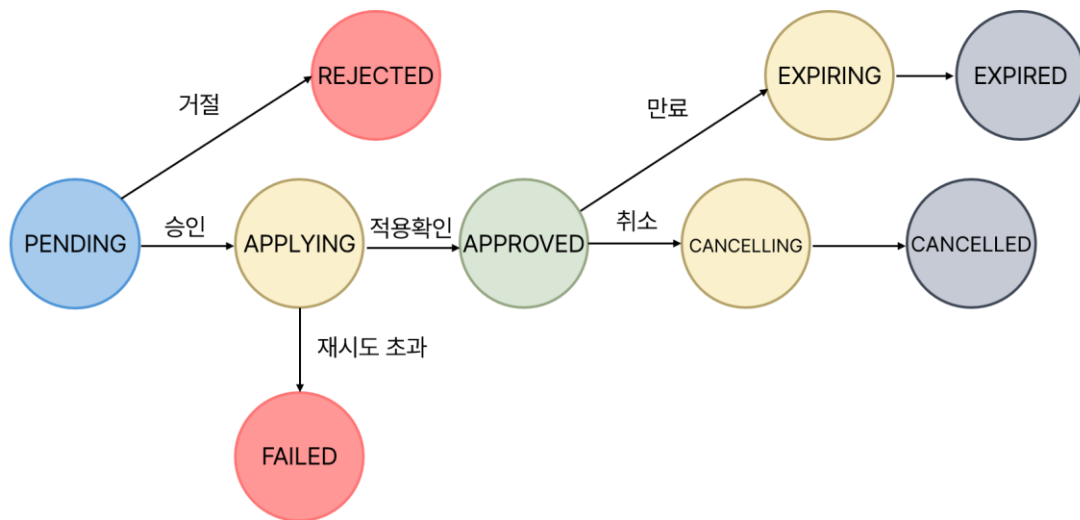
그림 2. 예외 요청 생명주기 상태 전이
