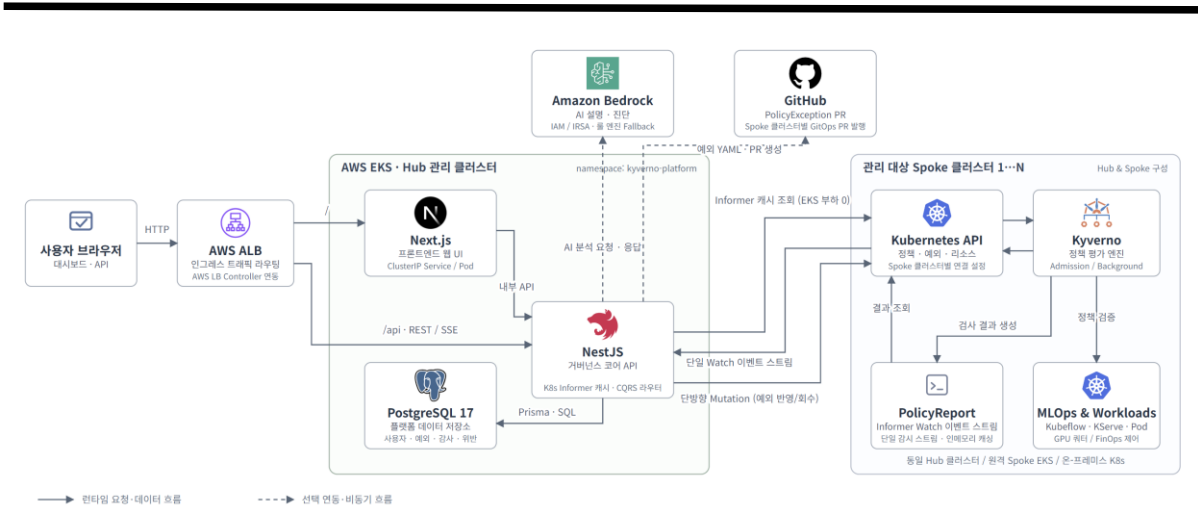
그림 1. 시스템 전체 구조
