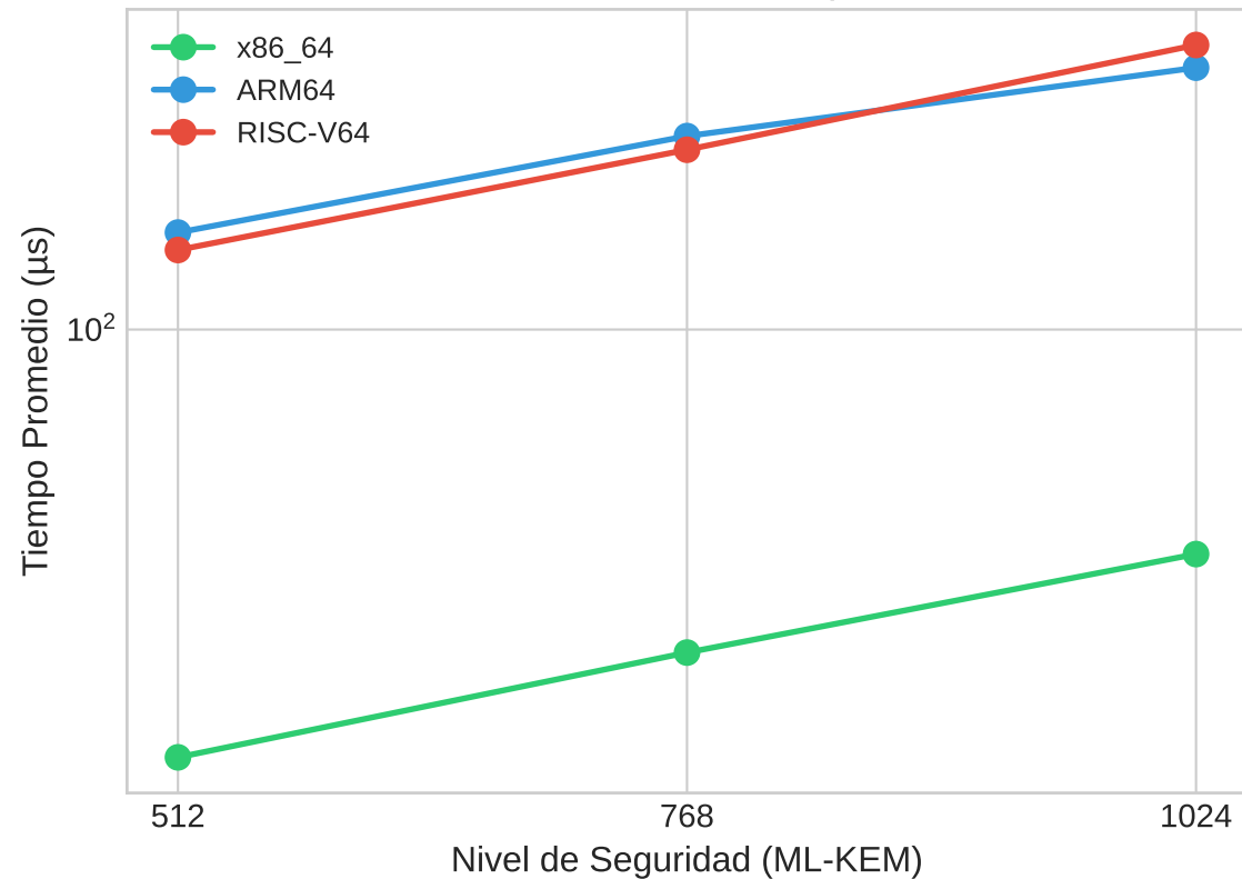
ML-KEM: Escalamiento por Nivel
