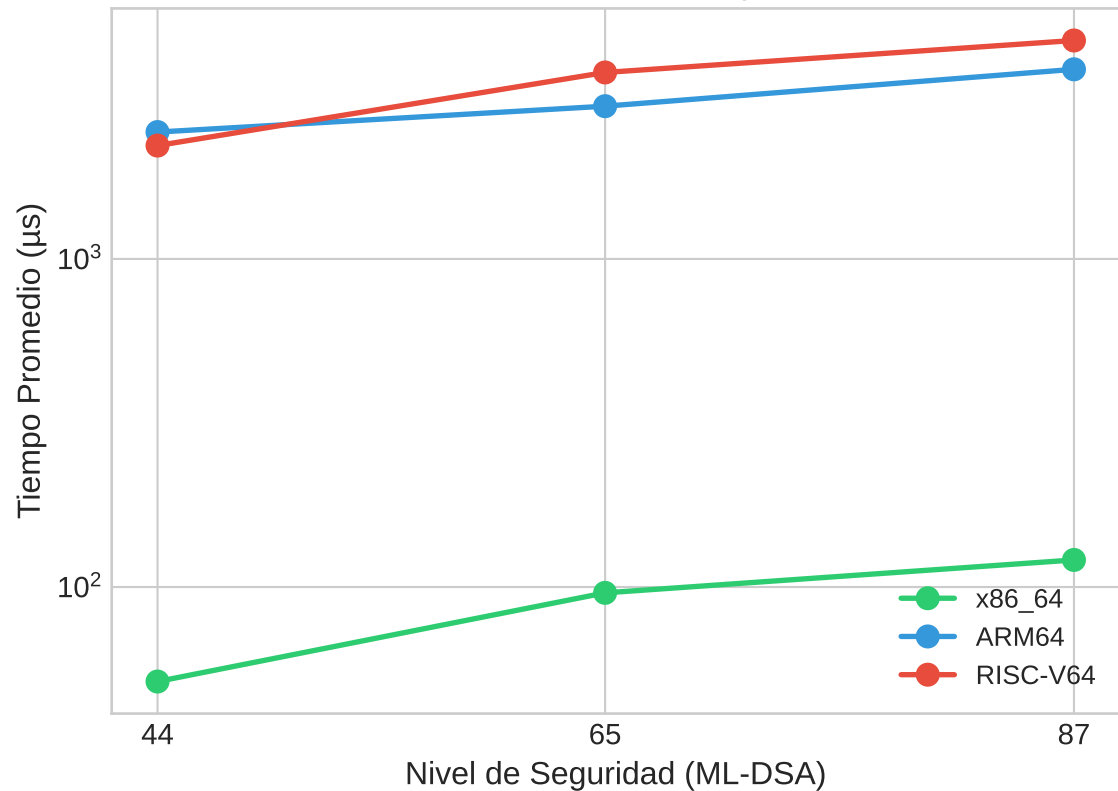
ML-DSA: Escalamiento por Nivel
