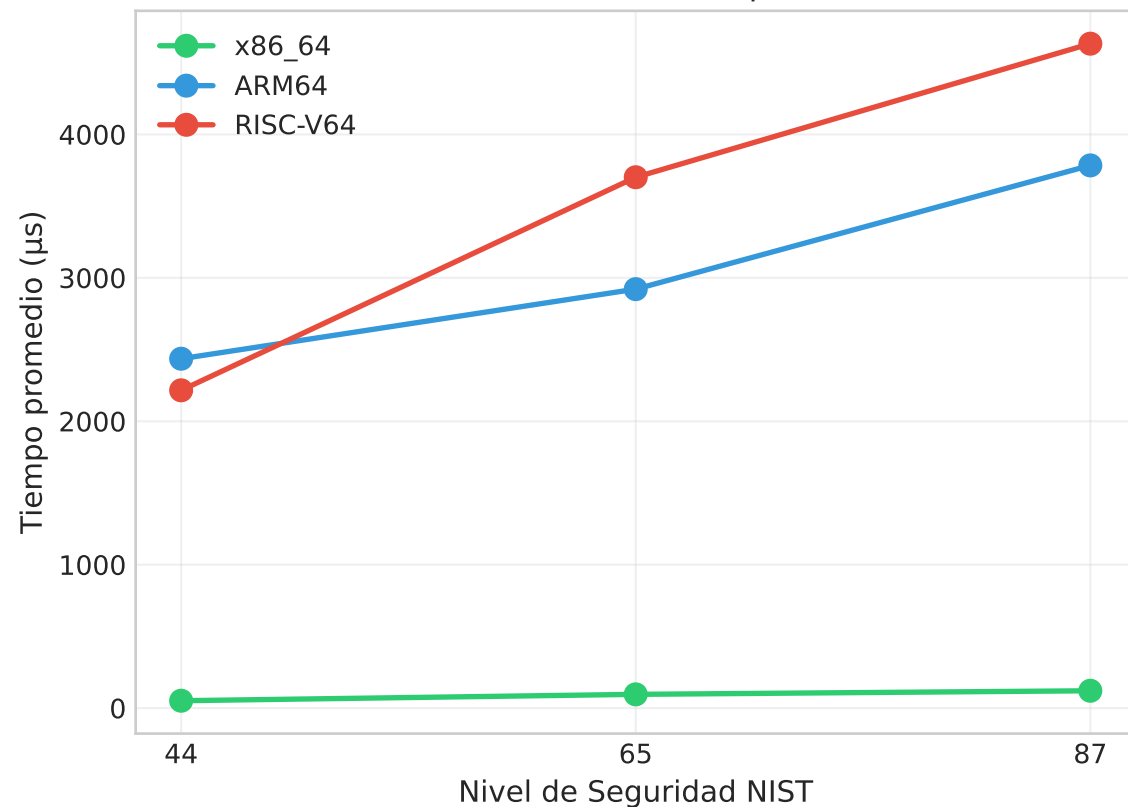
ML-DSA: Escalamiento por Nivel
