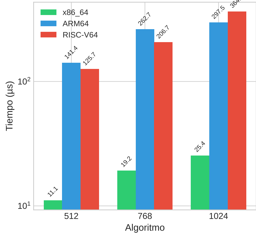
ML-KEM KeyGen
