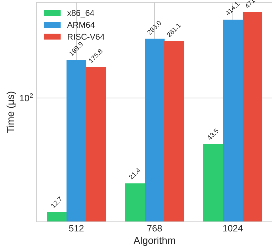
ML-KEM Decaps
