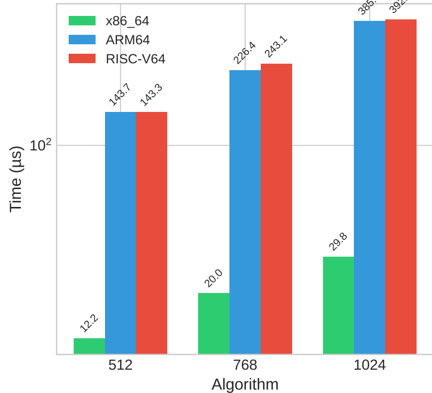
ML-KEM Encaps
