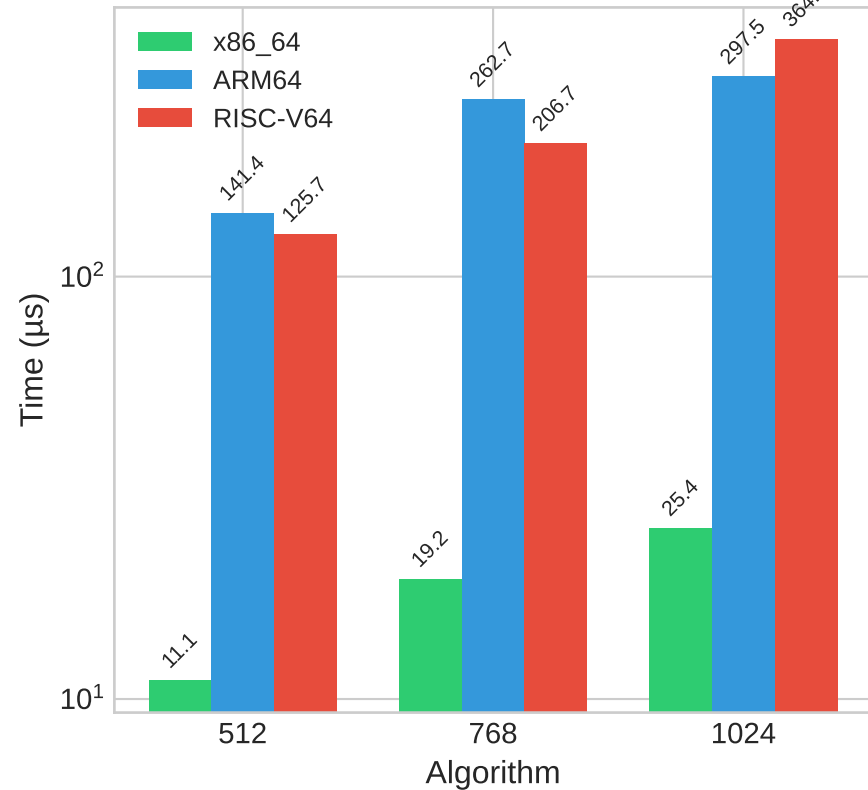
ML-KEM KeyGen
