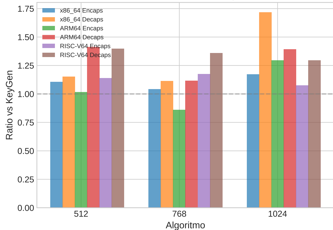
ML-KEM: Costo Relativo de Operaciones
