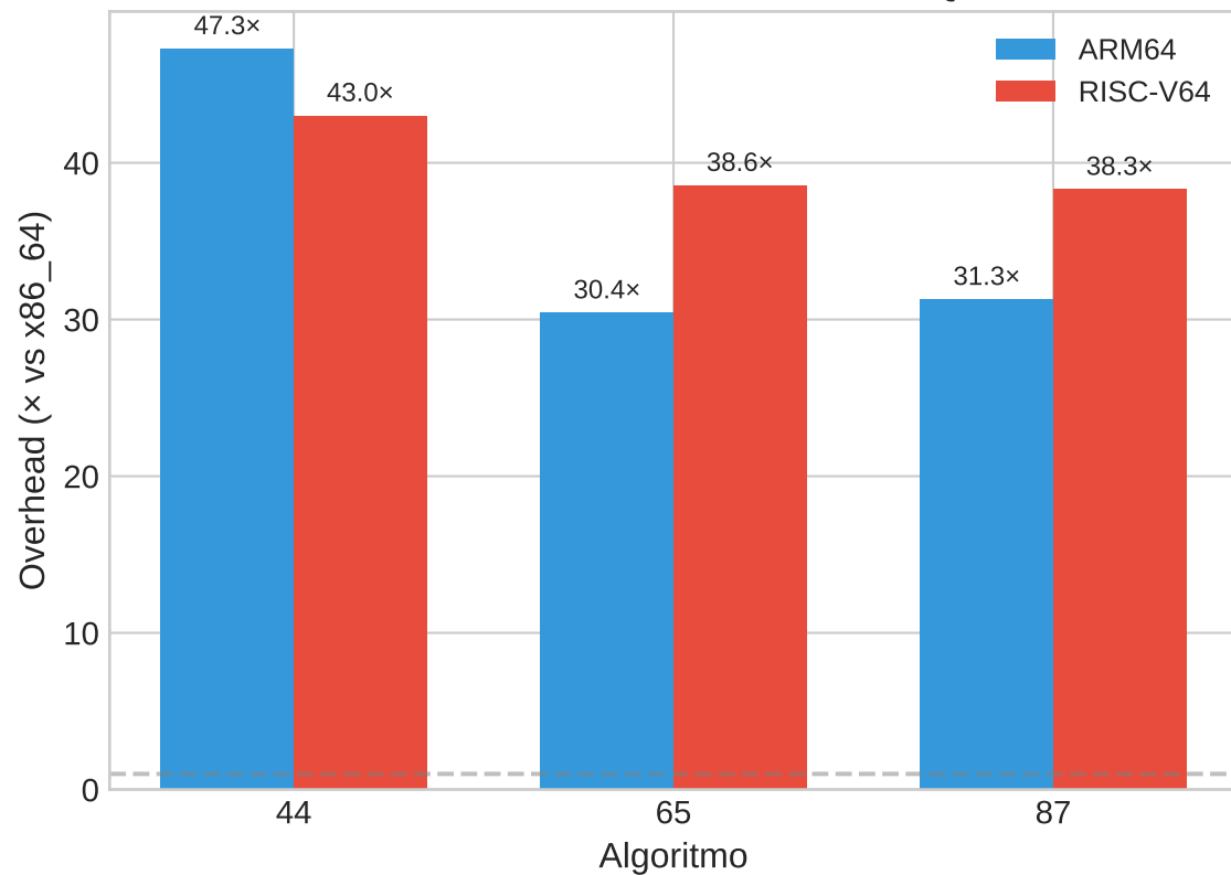
ML-DSA: Overhead de Emulación QEMU
