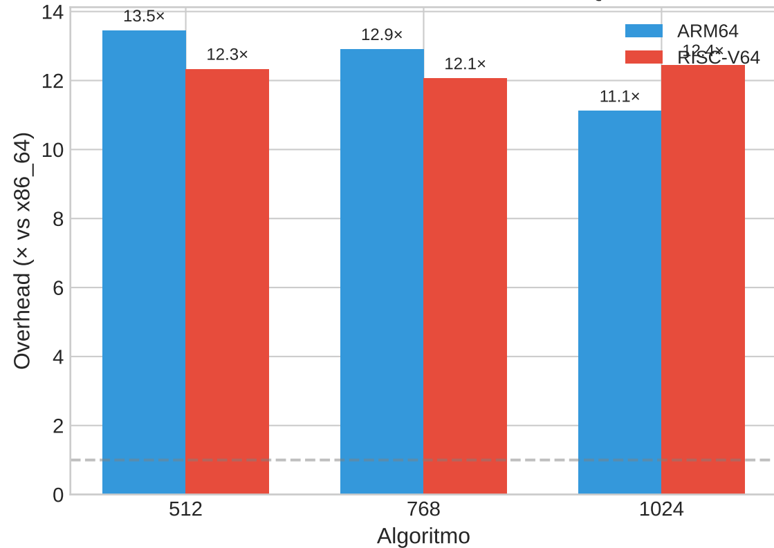
ML-KEM: Overhead de Emulación QEMU
