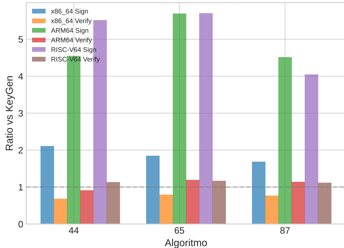
ML-DSA: Costo Relativo de Operaciones
