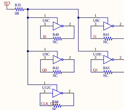
輸出Buffer - 負回饋電路 (SN74LVC1404DCUR)
