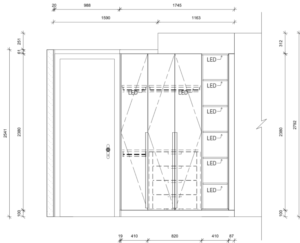
ELEVATION A
