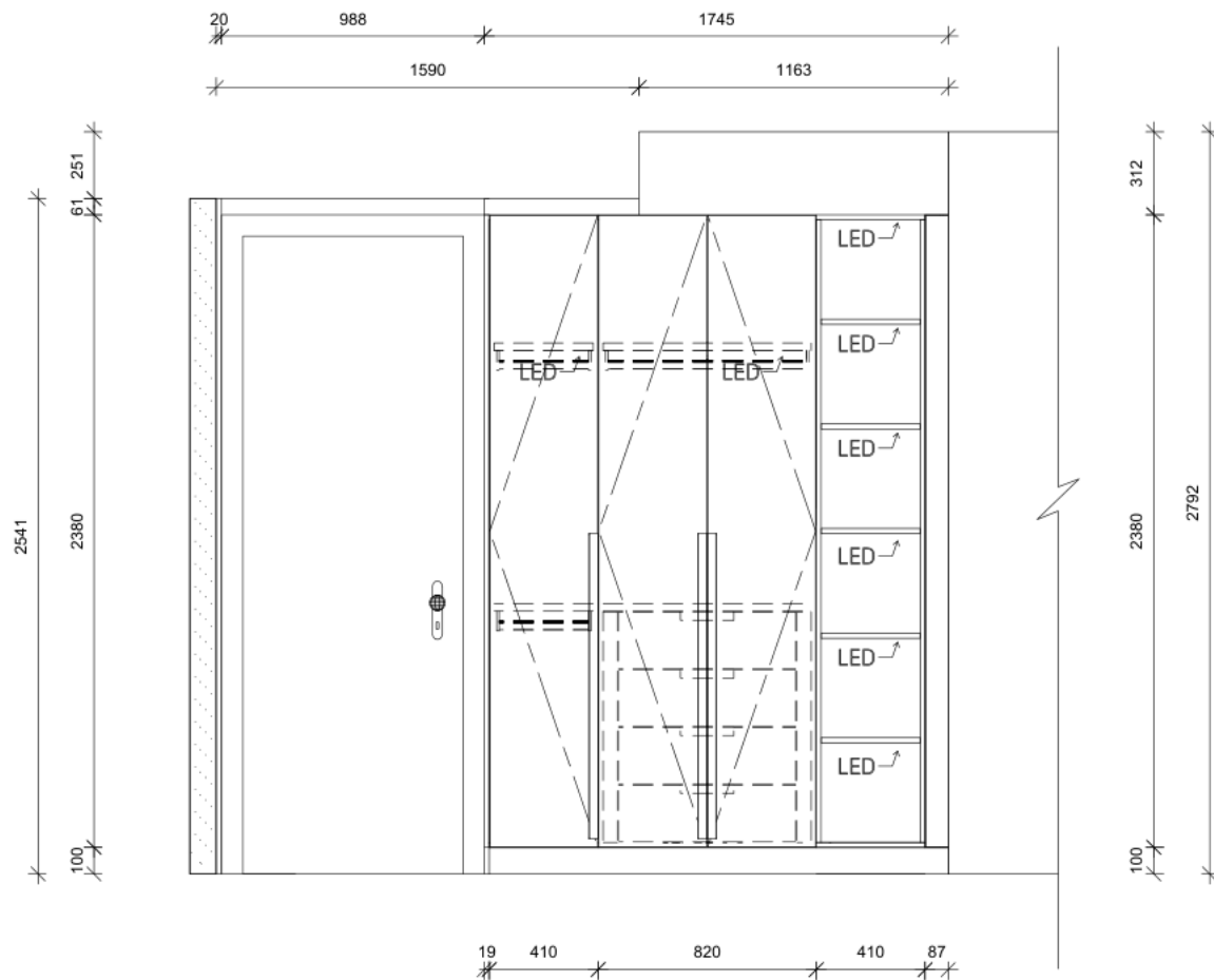
ELEVATION A
