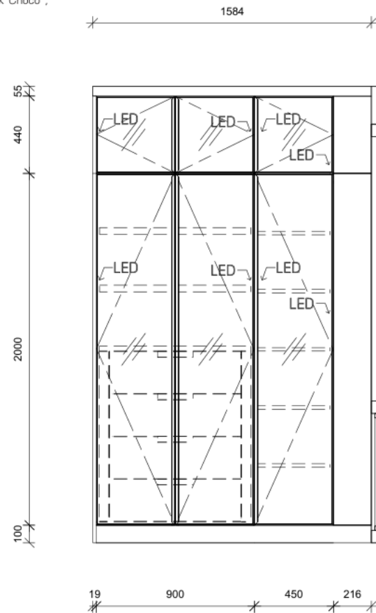
ELEVATION B
