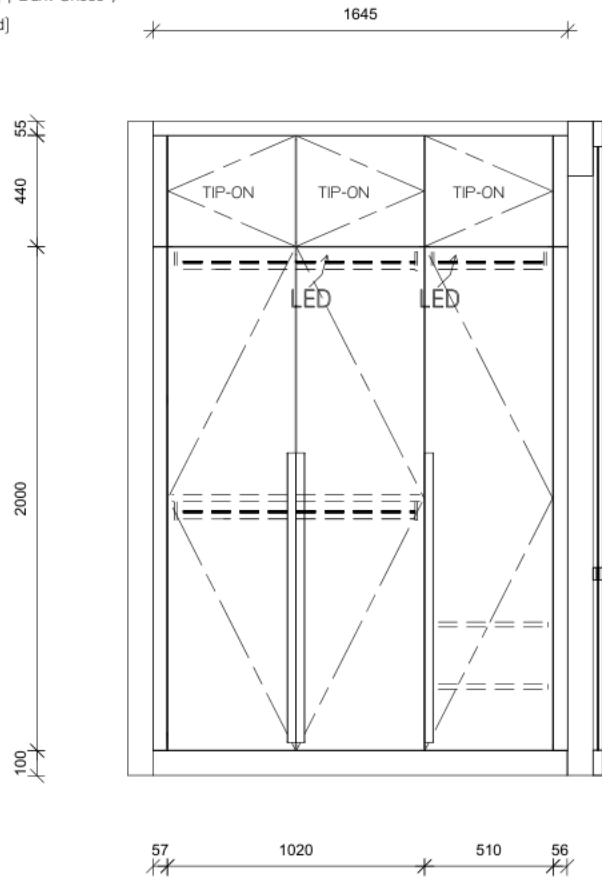
ELEVATION A
