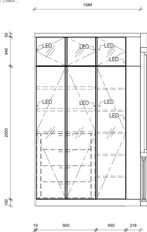
ELEVATION B
