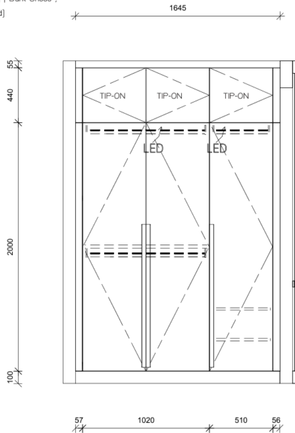
ELEVATION A
