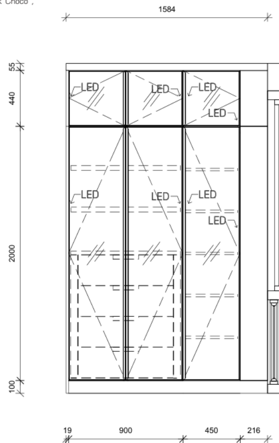
ELEVATION B
