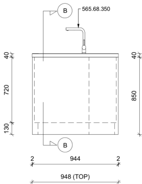
ELEVATION B
