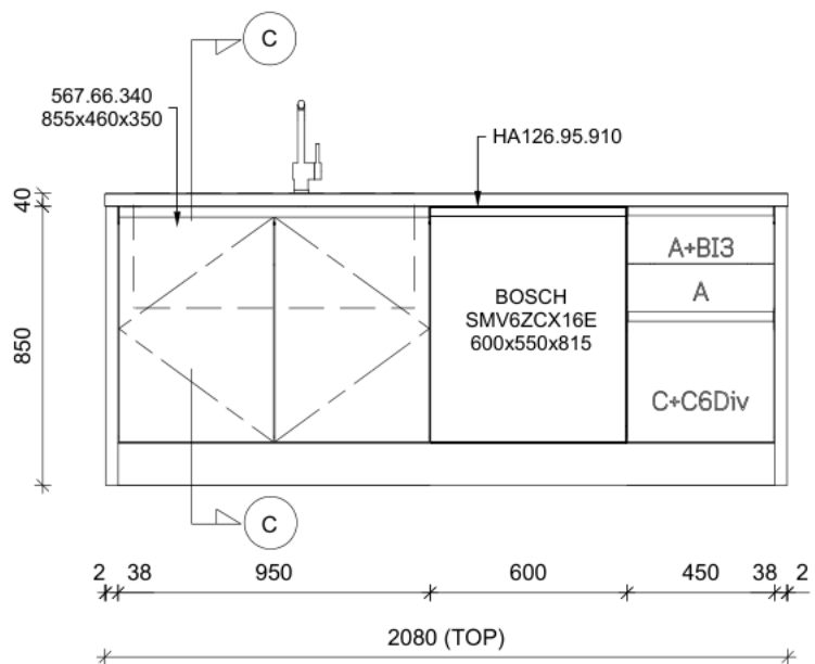
ELEVATION A
