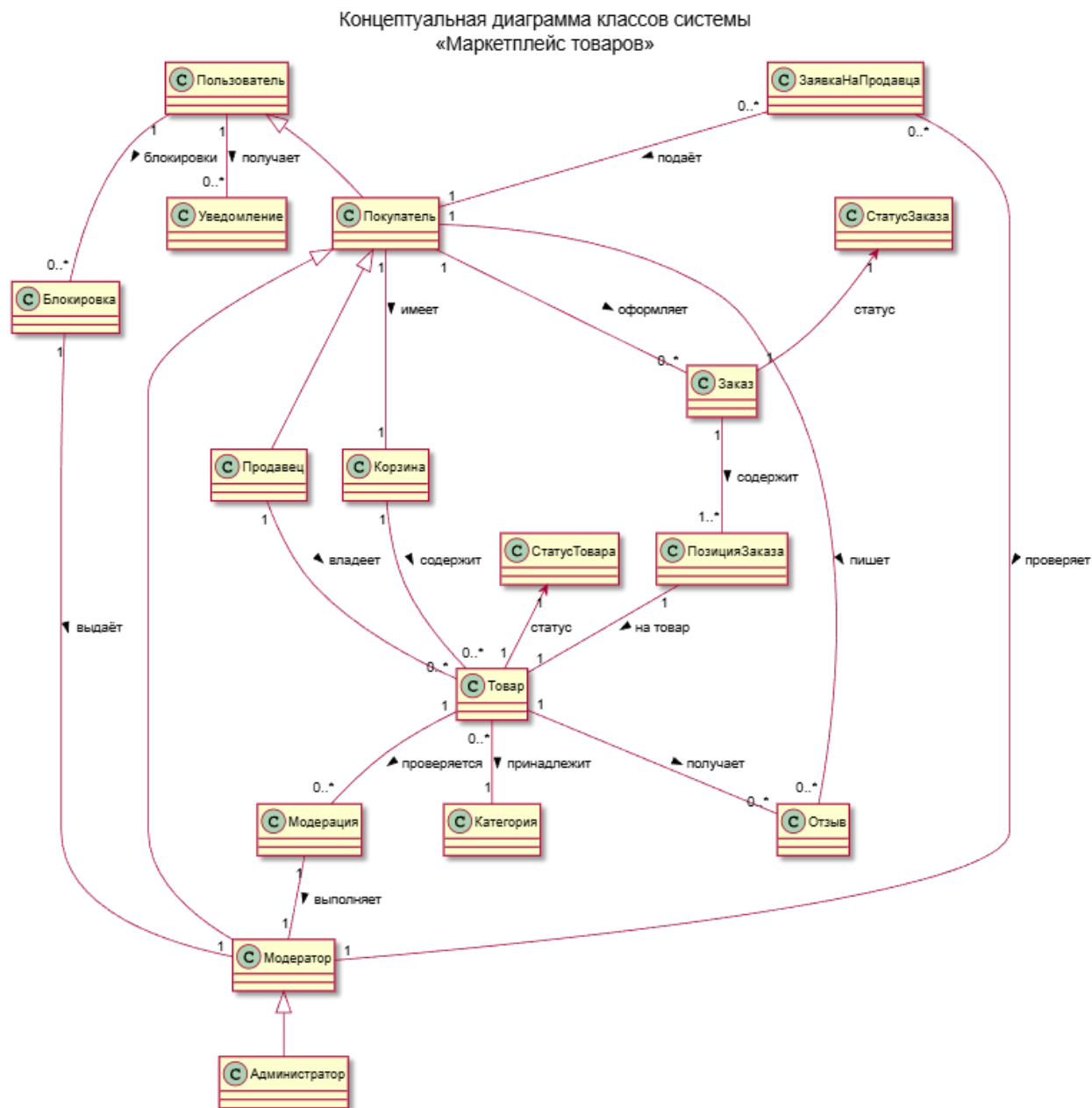
Рисунок 4 – Концептуальная диаграмма классов.
