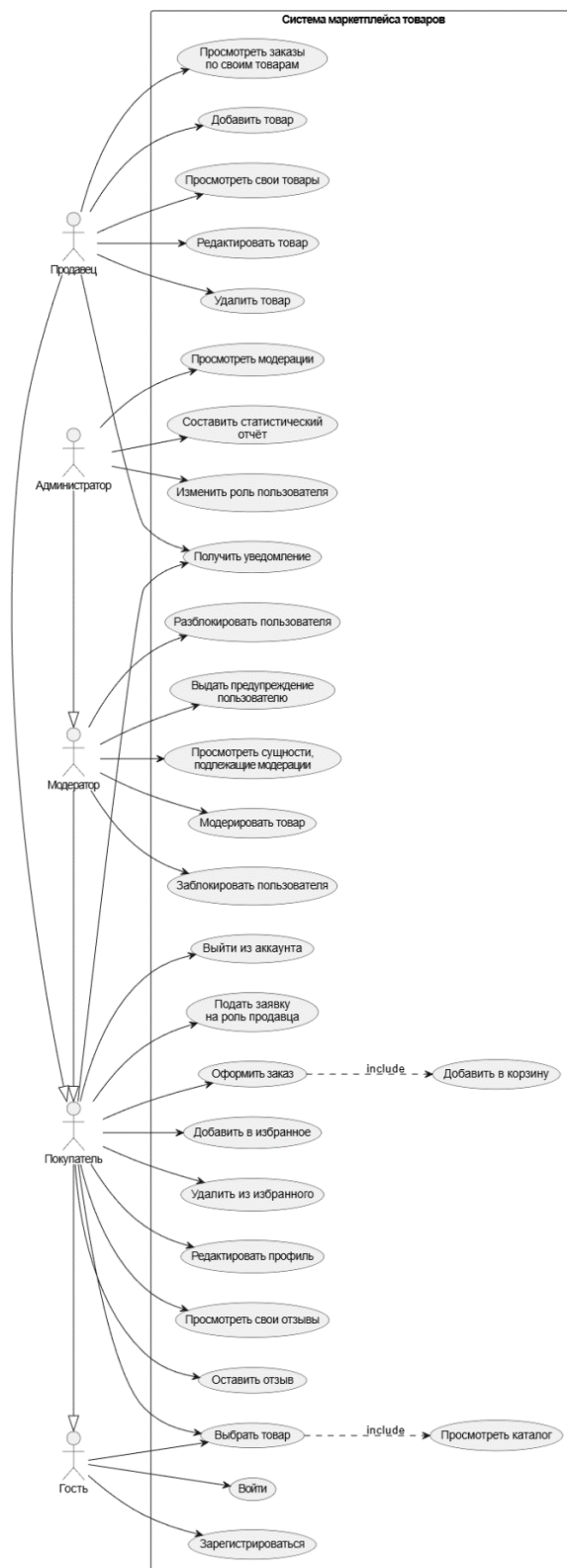
Рисунок 3 – Диаграмма прецедентов.
