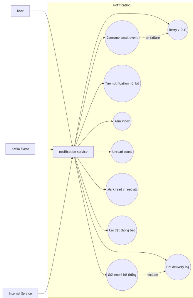
Hình 3.1: Sơ đồ use case chi tiết Notification Service
