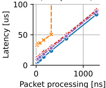
(d) Latency (64B packets)
