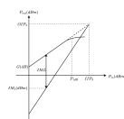
图 1.1: OIP3 与 IIP3 的关系
