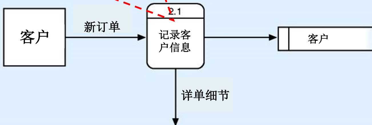
处理2.1（记录客户信息）和它的结构化语言描述
