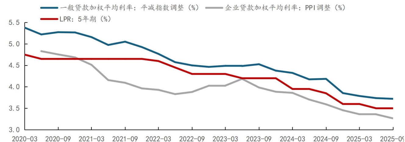
图表 3：社会实际利率与 5 年期 LPR 走势
