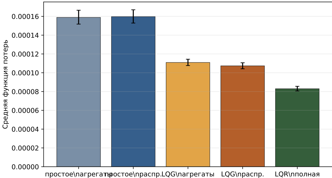
LQG/LQR-ориентир для совместной линейной системы
