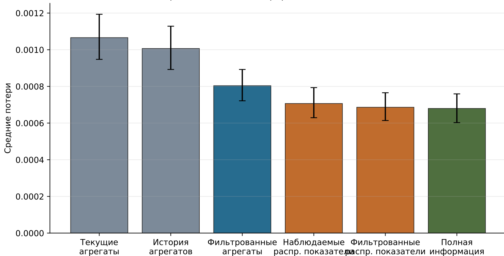
Потери политики по информационным состояниям
