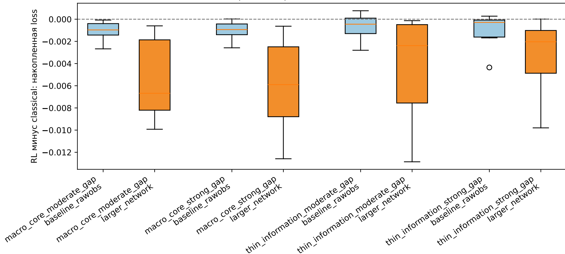
Разброс выигрыша RL по evaluation seeds
