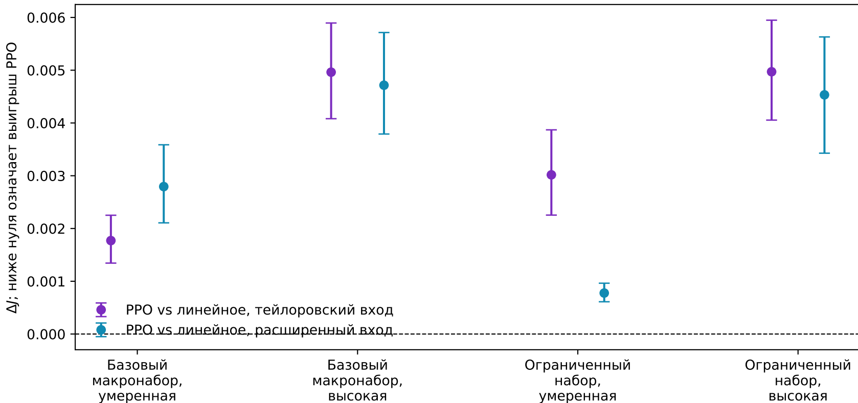
Same-input сравнение PPO и линейных baseline'ов
