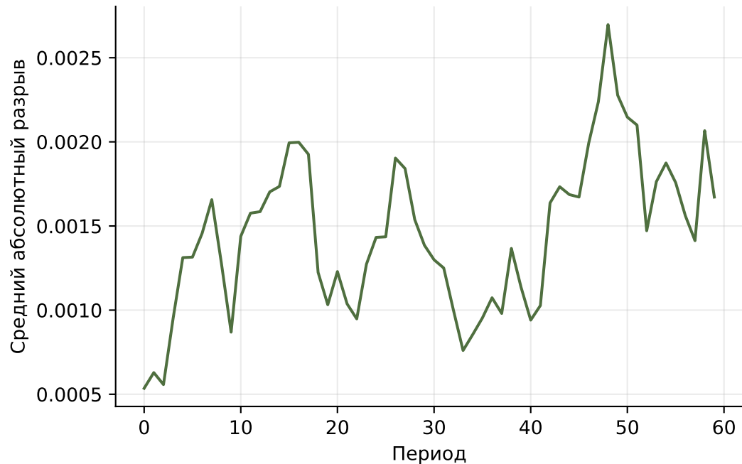
Разрыв выпуска на выигрышных траекториях
