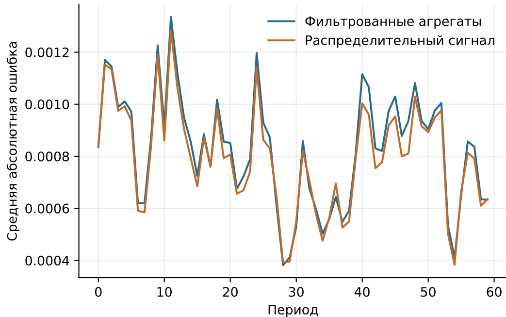
Ошибка предсказания оптимальной ставки
