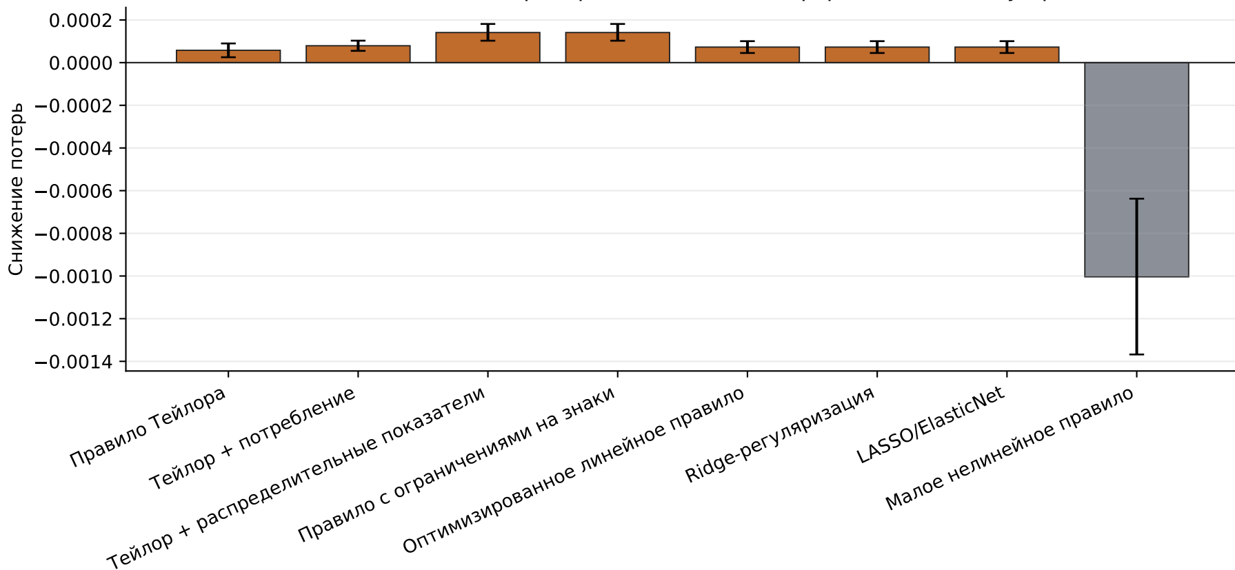
Устойчивость ценности распределительной информации к классу правила
