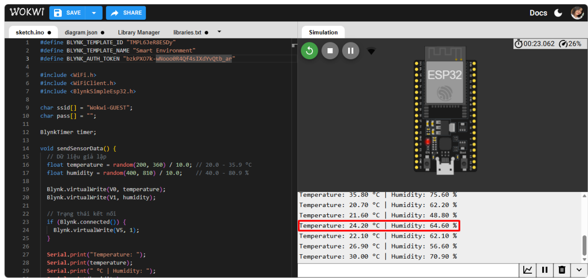
Hình BTVN1.2. Wokwi ESP32 gửi dữ liệu cảm biến lên Blynk
