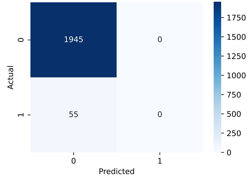
KNN
