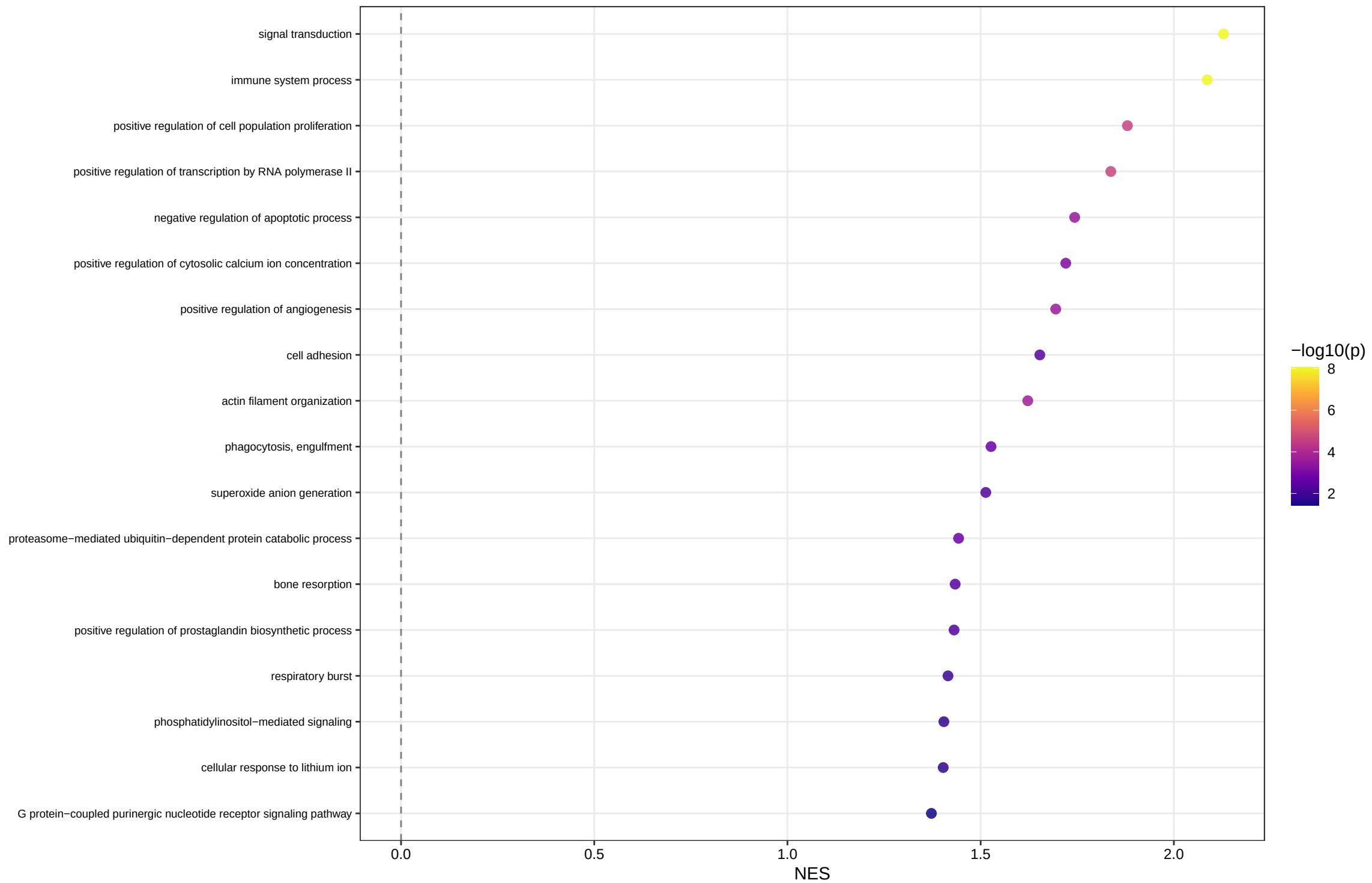
GO:BP GSEA – E2F (18 terms)
