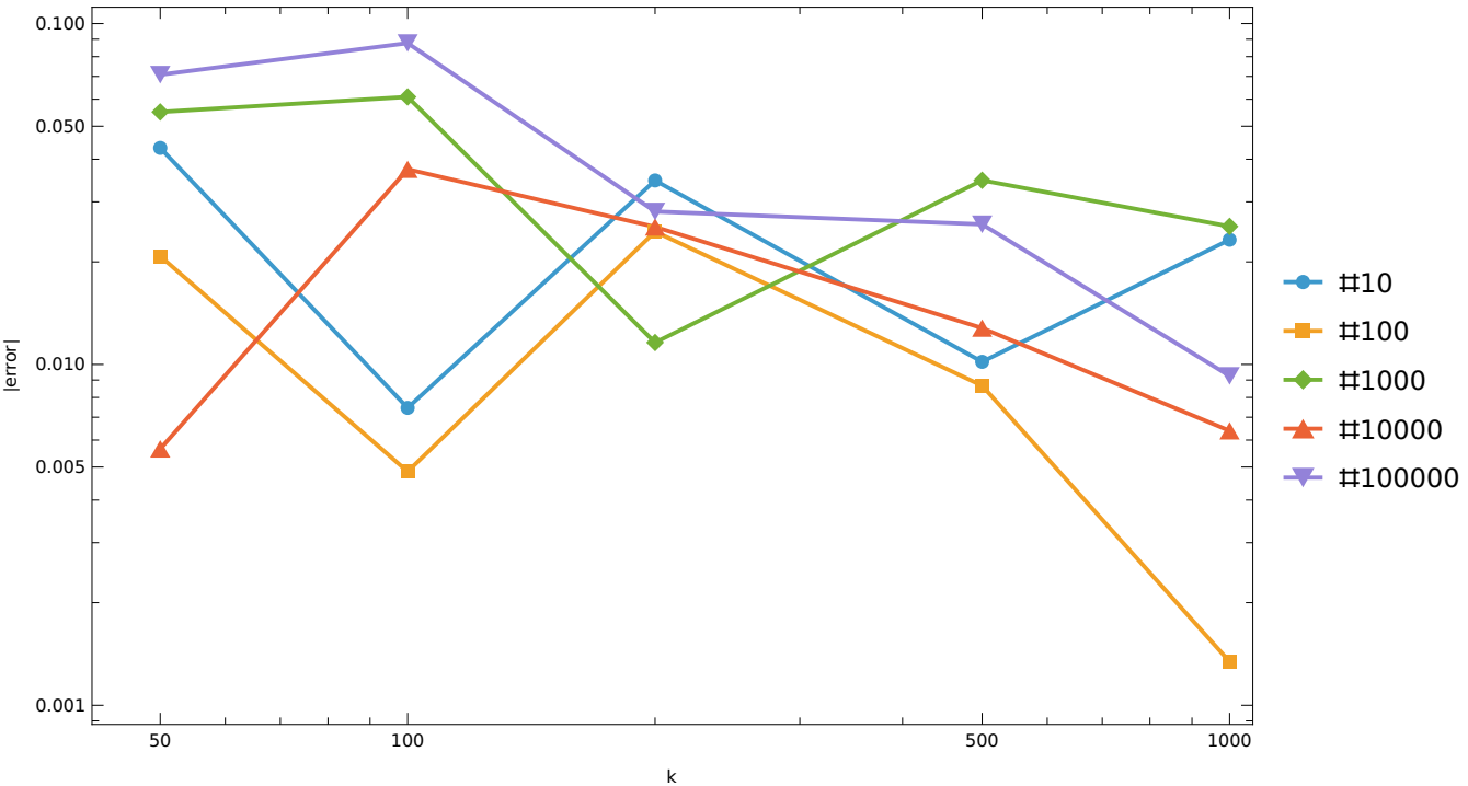
GHY B: finder error vs k
