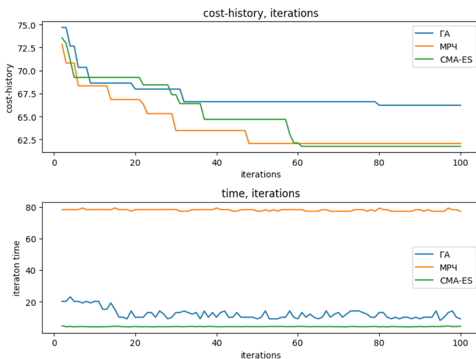
Рис.4.13. График изменения значения ЦФ по итерациям
