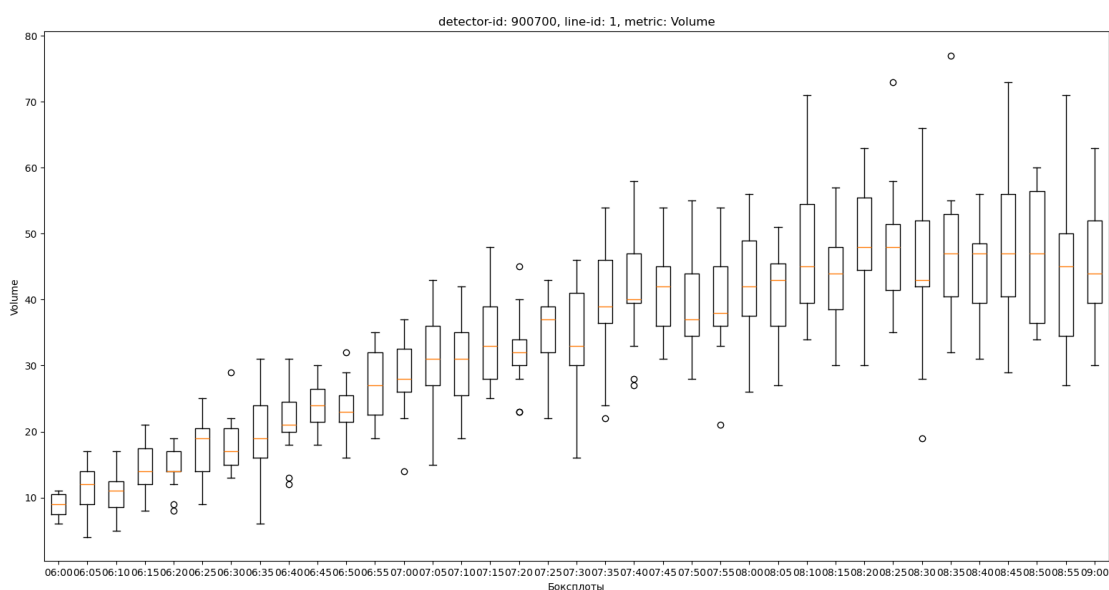
Рис.4.9. Боксплоты, отображающие среднюю интенсивность трафика по вр. интервалам, будни
