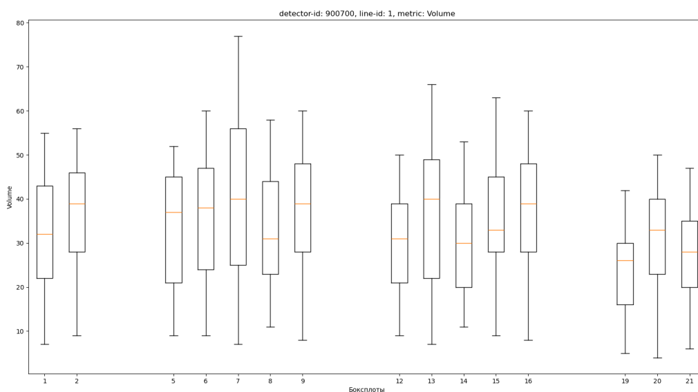
Рис.4.11. Боксплоты, отображающие среднюю интенсивность трафика по дням, будни
