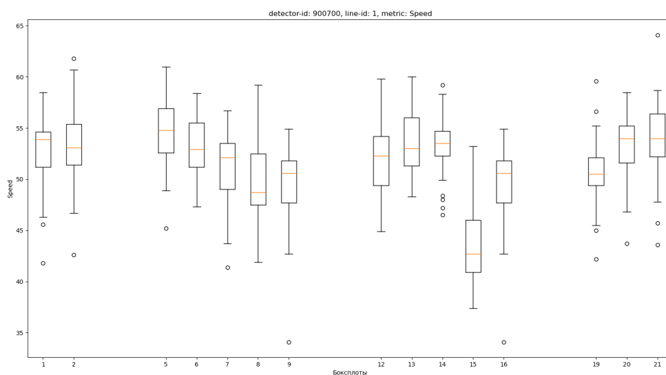
Рис.4.12. Боксплоты, отображающие среднюю скорость трафика по дням, будни
