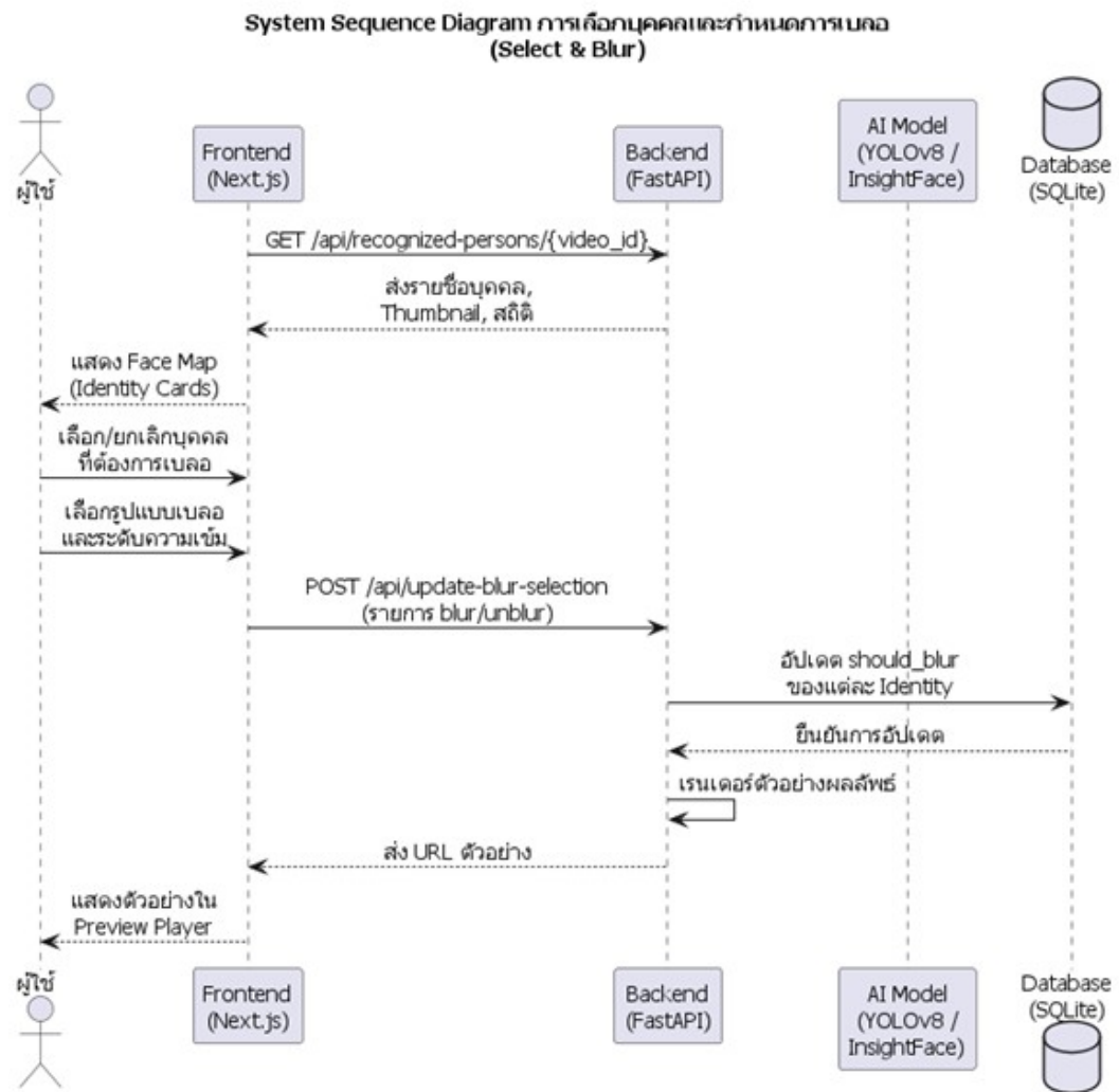
ภาพที่ 17 System Sequence Diagram การเลือกบุคคลและการปิดแบบรายบุคคล คำอธิบายภาพที่ 17: แสดงลำดับการโหลด Face Map การเลือกบุคคลและรูปแบบการปิด การบันทึกค่า should_blur และการสร้างตัวอย่างตามตัวเลือกของผู้ใช้
