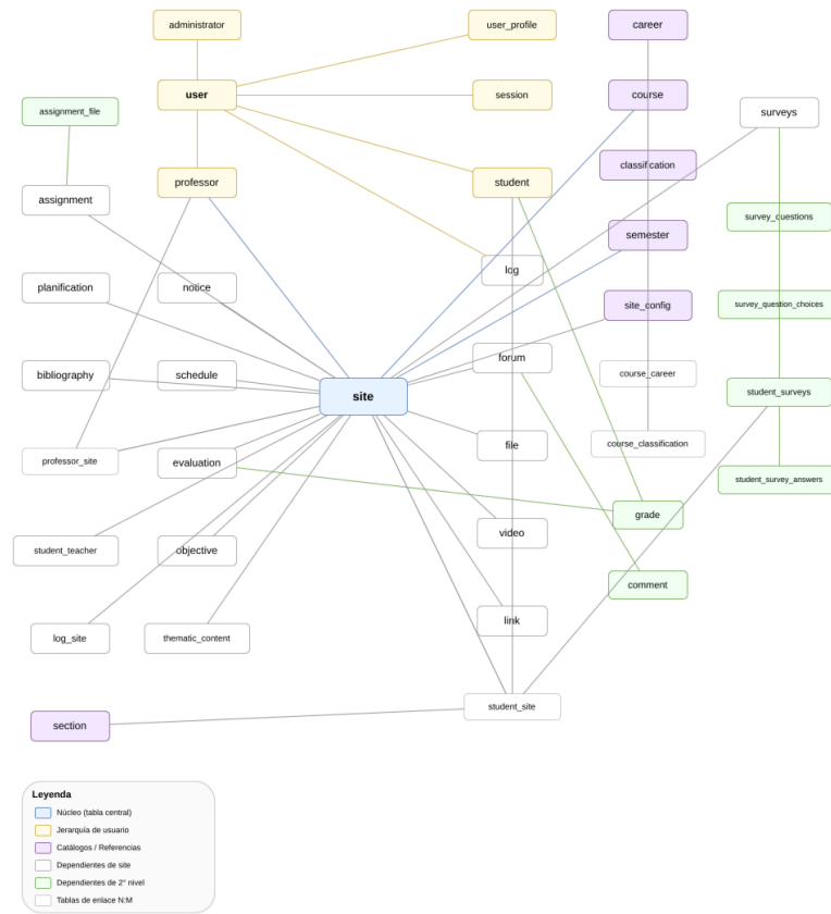
Figura 3.1: Diagrama entidad-relación simplificado del modelo de datos monolítico, mostrando la tabla site como núcleo con sus 15+ relaciones hacia entidades dependientes.
