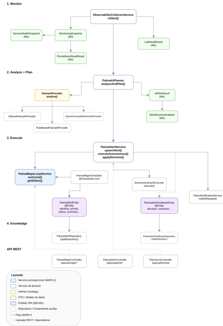
Figura 3.6: Diagrama de clases de PAIMA mostrando los paquetes del ciclo MAPE-K.
