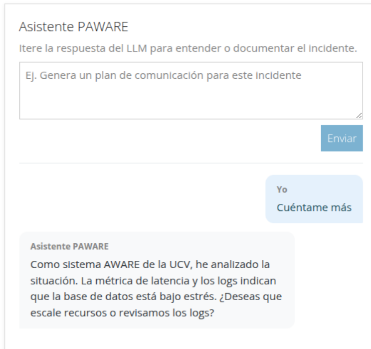
Figura 3.9: Interacción del administrador con el agente de IA para refinar el diagnóstico antes de ejecutar una acción sobre la alerta.
