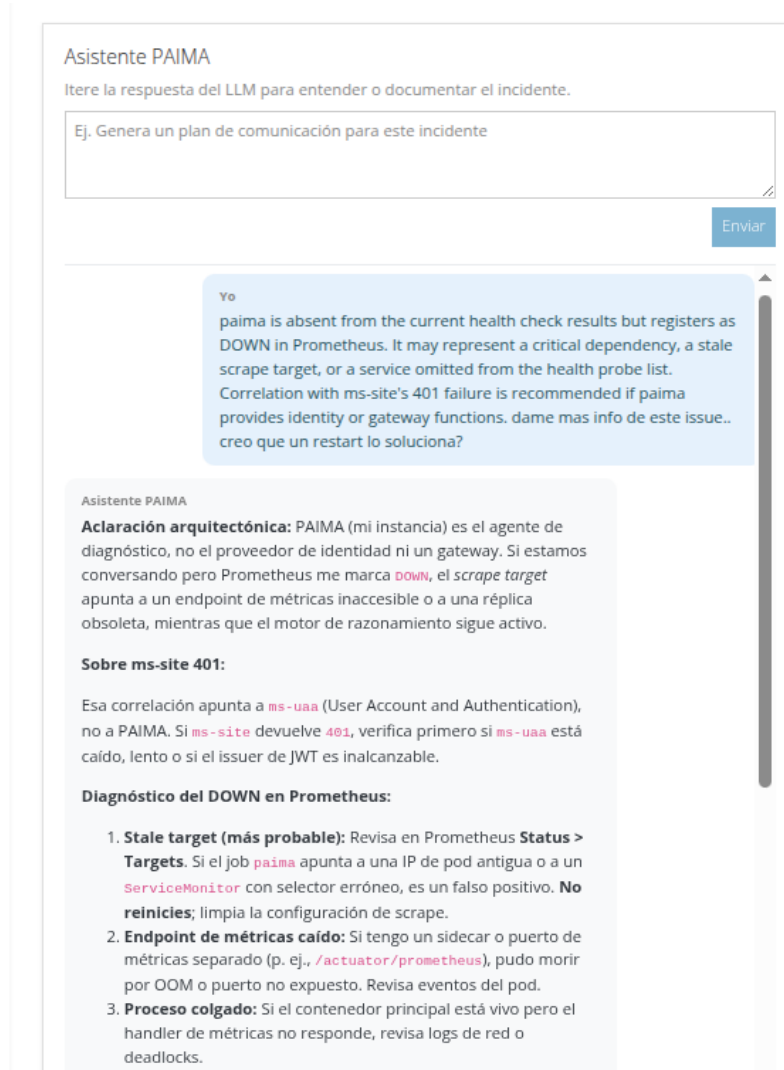
Figura 4.11: Interacción del administrador con el agente de IA para refinar el diagnóstico.
