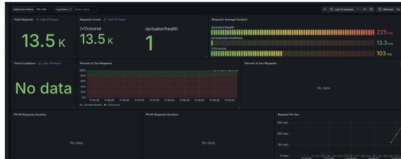
Figura 3.6: Exploración de logs con Grafana y Loki durante el arranque del ecosistema de microservicios.
