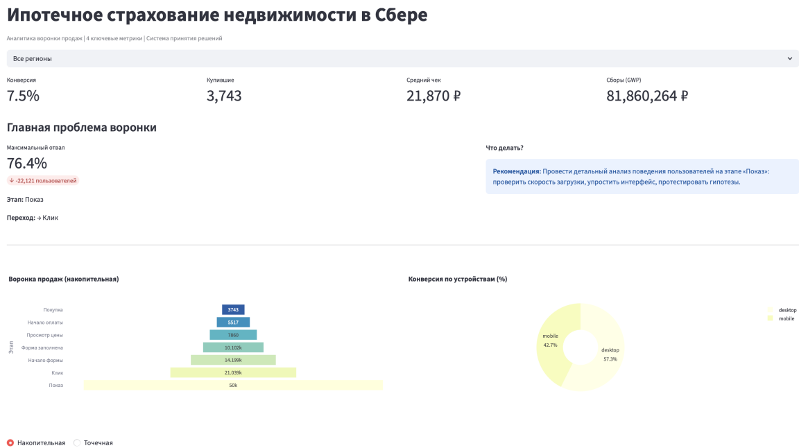
Рис. 1: Интерфейс дашборда
