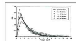
그림 2. 밀의 배출에서 고체 백분율이 다른 밀 반자동 시험용 밀의 DTR 곡선 및 완벽한 혼합 모델 조정.
